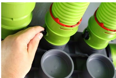
Regulace na rozdělovacím DBoxu pomocí regulačních klapek
